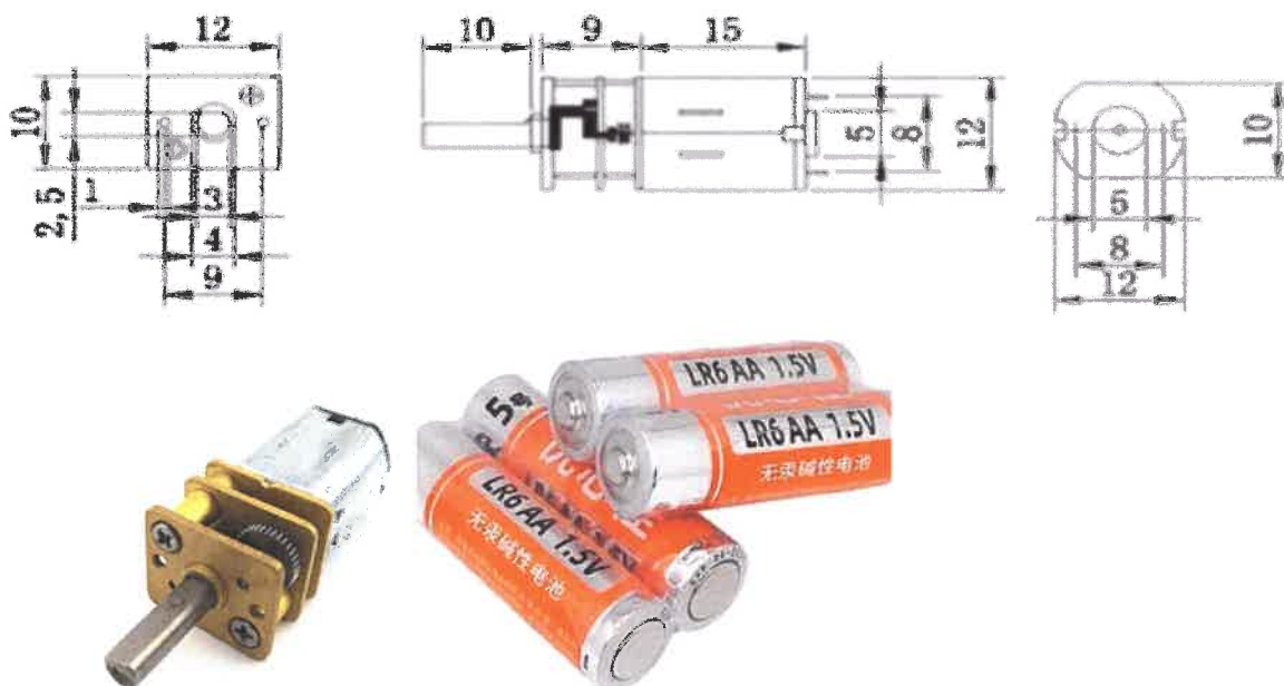
图 3 电动机、电池外观（供参考）
